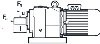
Çıkış Milinde Radyal Kuvvet Hesabı Düzeltme Katsayıları
